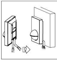
Monté à plat plana
