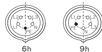
Fig: frontal de ficha ou tomada fêmea
